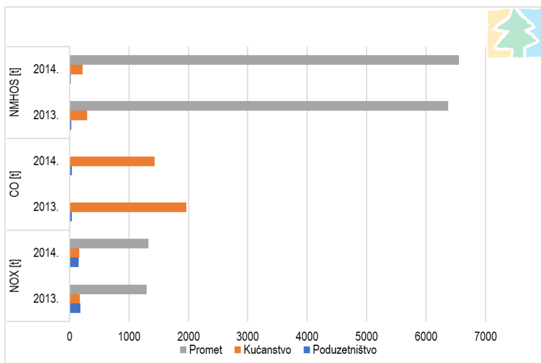
Slika 4.19 Usporedba emisija NO x , CO i NMHOS iz sektora prometa, kućanstva i poduzetništva Županije u 2013. i 2014. godini (Izrađivač: IRES EKOLOGIJA d.o.o.)
