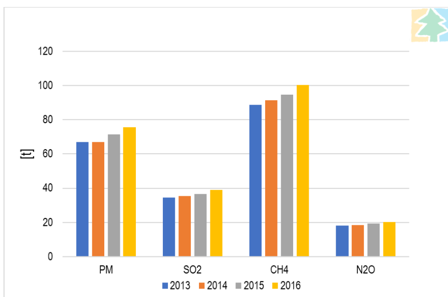
Slika 4.15 Ukupne emisije PM, SO 2 CH 4 i N 2 O iz cestovnog prometa u razdoblju od 2013. do 2016. godine na području Županije (Izrađivač: IRES EKOLOGIJA d.o.o.)
