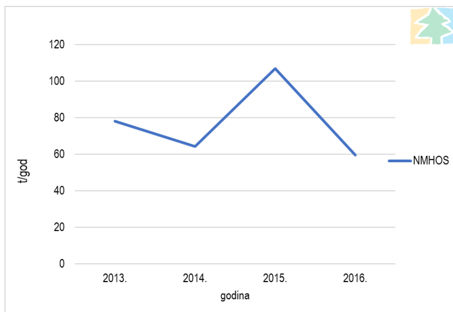
Slika 4.10 Procijenjene emisije NMHOS iz otpada na području Županije u razdoblju od 2013.-2016. godine (Izrađivač: IRES EKOLOGIJA d.o.o.)
