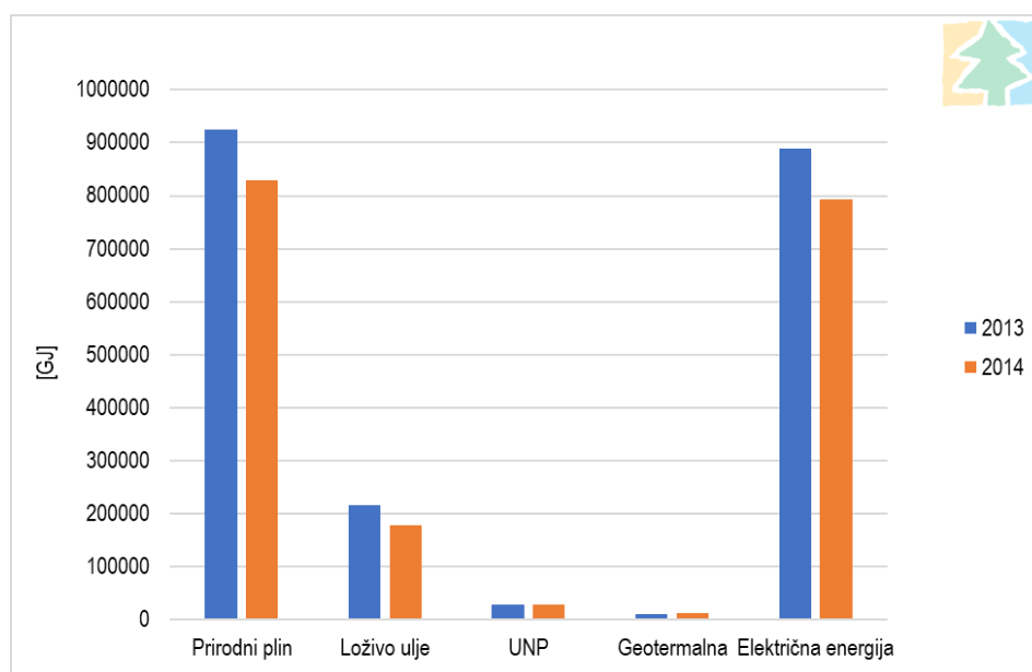
Slika 4.5 Ukupna potrošnja energije u sektoru poduzetništva Županije u 2013. i 2014. godini (Izvor: APEnU)
