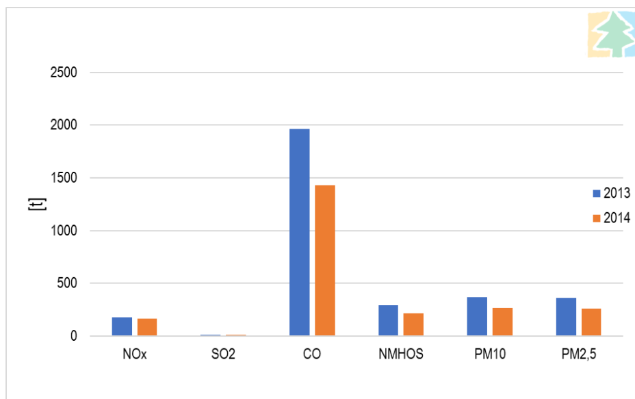
Slika 4.8 Emisija pojedinih onečišćujućih tvari iz sektora kućanstva u 2013. i 2014. godini na području Županije (Izradivač: IRES EKOLOGIJA d.o.o.)
