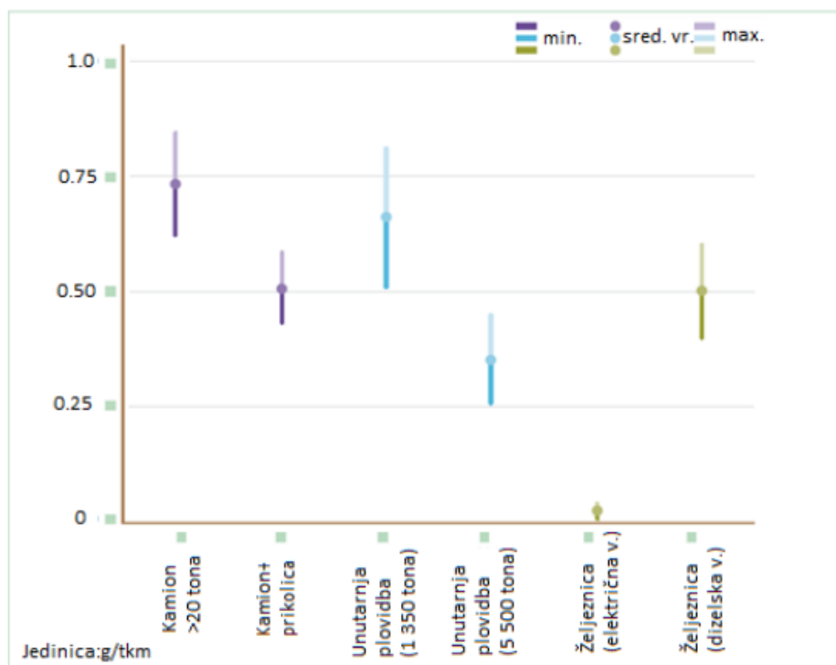
Slika 4.17 NOx emisija kod teretnog prijevoza u 2010. godini na dugim udaljenostima (> 150 km); (Izvor: The power of inland navigation; Diplomski rad: Marko Čikširan)
