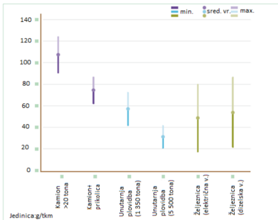
Slika 4.16 Emisija CO 2 kod teretnog prijevoza u 2010. godini na dugim udaljenostima (>150 km) (Izvor The power of inland navigation; Diplomski rad: Marko Čikširan)
