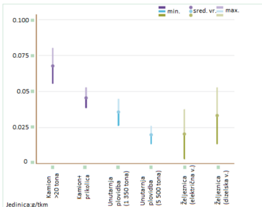
Slika 4.18 SO2 emisija kod teretnog prijevoza u 2010. godini na dugim udaljenostima (> 150 km); (Izvor: The power of inland navigation; Diplomski rad: Marko Čikširan)
